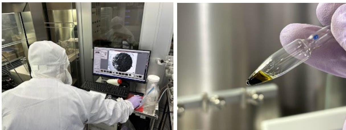
図 2. 左：九州大学大学院理学研究院 地球惑星科学部門のクリーンルーム実験室における分析の模様。 右：塩酸とともに加熱したベヌー試料。
