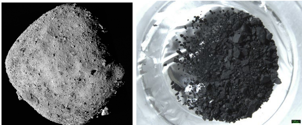
図 1. 小惑星ベヌー（左。©NASA）と分析に用いた試料（OREX-800044-101）の光学顕微鏡写真（右）。スケールバーは 500 \mu\text{m} 。
